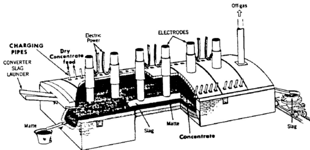
Horno eléctrico cerrado de arco
