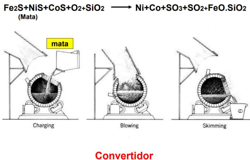
Figura 5: Esquema de un convertidor Peirce-Smith.
